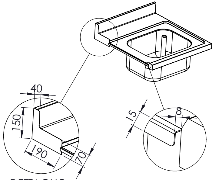
DETTAGLIO SCALA 1 : 10
